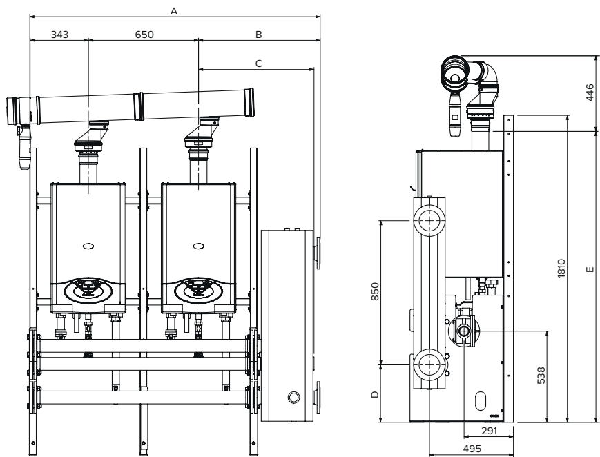
КОЛЕКТОРИ DN65
