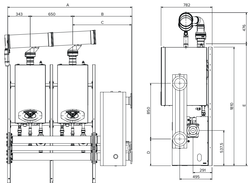
КОЛЕКТОРИ DN100
